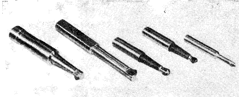
Рис. 2.4. Расточные резцы для координатно-расточных станков, оснащенные композитом 01 или 10
