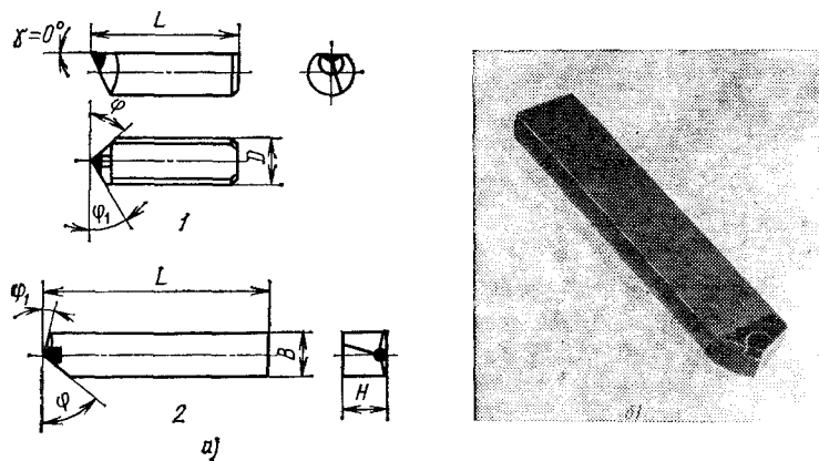
Рис. 2.3. Расточные резцы, оснащенные композитом 01 или 10: а — конструкция; 1 — круглого сечения; 2 — прямоугольного сечения; б — общий вид
