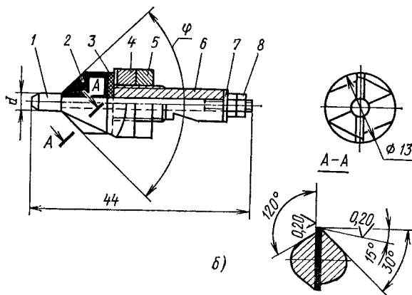
Рис. 2.17. Зенковка с механическим креплением пластин из композита 05: а — общий вид; б — конструкция d = 3 \dots 6 мм; \varphi равно 90^\circ и 120^\circ ; 1 — направляющий штырь; 2 — специальная пятигранная перетачиваемая пластина из композита 05; 3 — демпфирующая шайба; 4 — корпус; 5 — контргайка; 6 — полый винт-хвостовик; 7 — шайба; 8 — гайка
