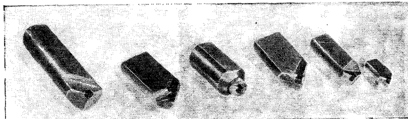
Рис. 2.1. Вставки резцовые с неразъемно закрепленным (запаянным) поликристаллом композитов 01, 02 или 10
