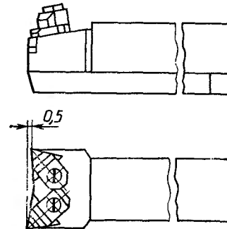
Рис. 2.26. Двусторонний токарный резец с пластинами из керамики для наружного точения и растачивания
