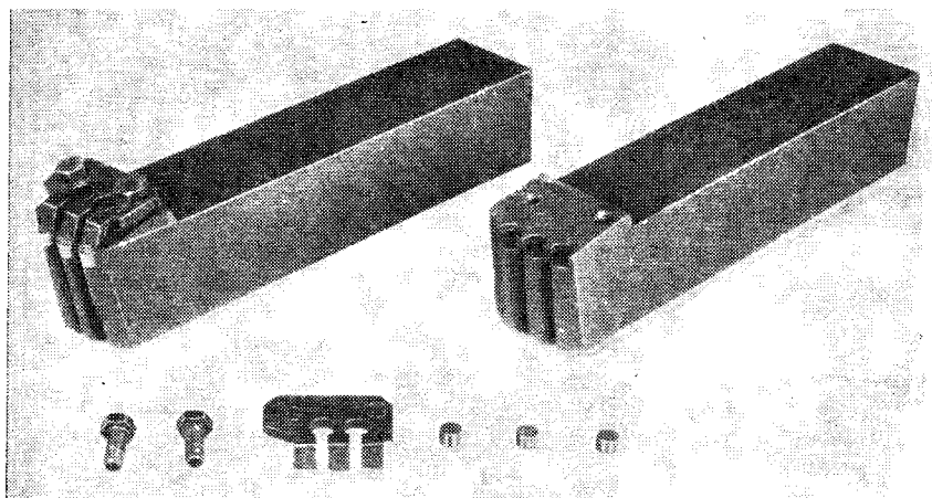
Рис. 2.9. Резец токарный ступенчатый для обработки прокатных валков
