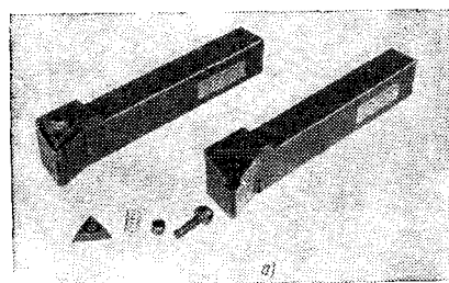
Рис. 2.6. Резец токарный сборный с механическим креплением пластин из композита (пластина базируется в закрытом гнезде в корпусе): а — общий вид; б — конструкция; 1 — пружина; 2 — режущая пластина из композита; 3 — крепежный винт; 4 — прихват; 5 — опорный выступ; 6 — корпус
