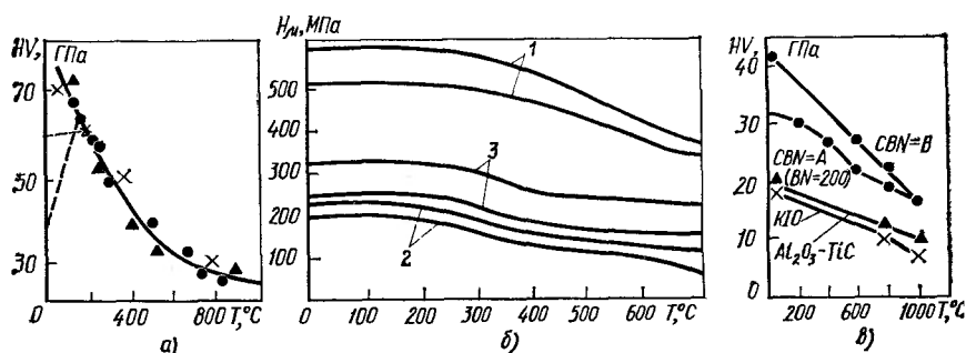
Рис. 1.2. Зависимость твердости HV поликристаллов на основе ВN от температуры:
