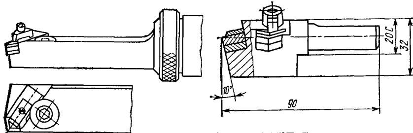
Рис. 2.29. Расточная оправка с пластинами из керамики для станков с ЧПУ
