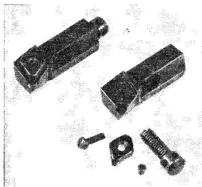
Рис. 2.8. Резцовая расточная регулируемая вставка с механическим креплением пластины из композита
