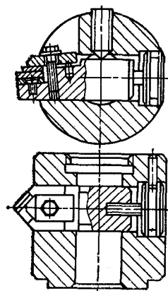
Рис. 2.28. Расточная головка с пластиной из керамики
