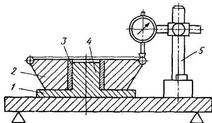
Рис. 2.12. Приспособление для настройки торцового биения ножей регулируемой фрезы вне станка:
