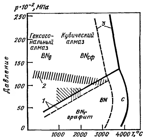
Рис. 1.1. Диаграмма состояния углерода и нитрида бора: 1 — линия равновесия слоистых и тетраэдрических фаз; 2 — линия равновесия прямых фазовых переходов; 3 — линия плавления
