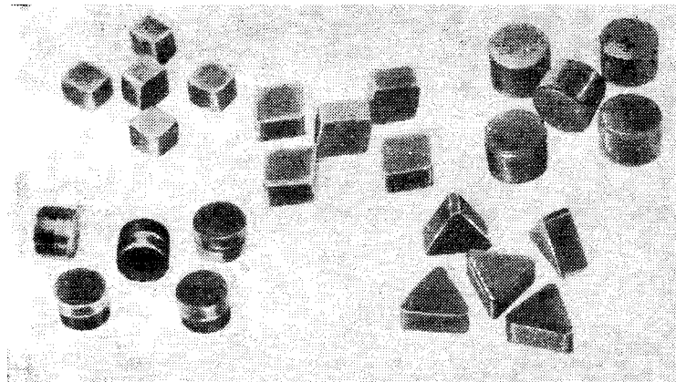
Рис. 2.5. Режущие цельные и двухслойные пластины из композитов
