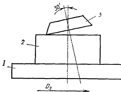
Рис. 2.16. Рекомендуемая схема фрезерования с наклоном шпинделя: 1 — стол станка; 2 — заготовка; 3 — фреза
