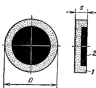
Рис. 2.18. Двухслойные заготовки для напайного инструмента:
