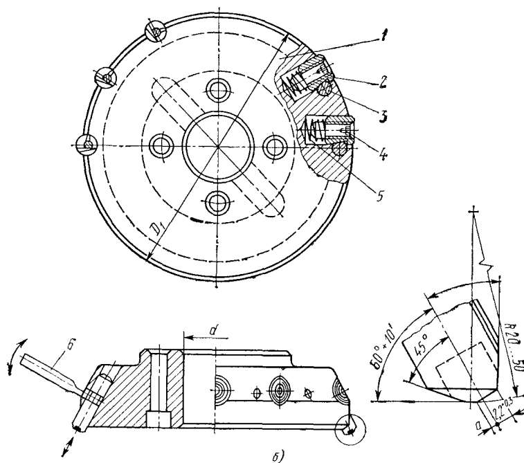
Рис. 2.11. Фреза торцовая насадная регулируемая со вставными перетачиваемыми ножами, оснащенными композитами О1 или 10: а — общий вид; б — конструкция
