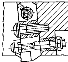
Рис. 2.34. Сборная торцовая фреза с регулируемыми вставками с пластинами из керамики фирмы «Фельдмюлле»
