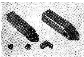
Рис. 2.7. Резцовая расточная вставка с механическим креплением ромбических пластин из композита:
