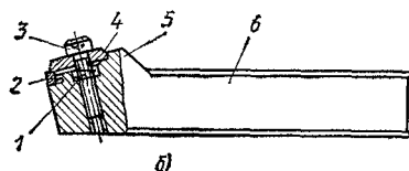
Рис. 2.6. Резец токарный сборный с механическим креплением пластин из композита (пластина базируется в закрытом гнезде в корпусе): а — общий вид; б — конструкция; 1 — пружина; 2 — режущая пластина из композита; 3 — крепежный винт; 4 — прихват; 5 — опорный выступ; 6 — корпус
