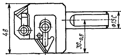
Рис. 2.29. Расточная оправка с пластинами из керамики для станков с ЧПУ
