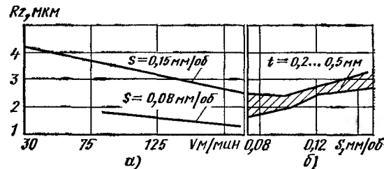
Рис. 3.2. Влияние скорости резания v при t = 0,5 мм (а) и подачи S_0 при v = 150 м/мин (б) на параметр шероховатости обработанной поверхности Rz
