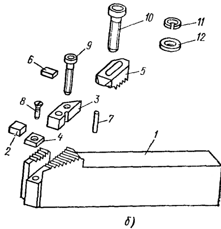
Рис. 2.25. Специальный токарный резец с пластинами из керамики: а — конструкция; б — конструктивные элементы
