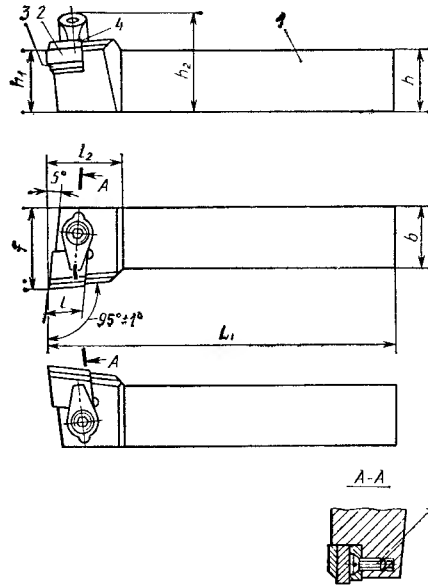
Рис. 2.21. Резец с механическим креплением ромбической пластины из керамики; 1 — державка; 2 — опорная пластина; 3 — режущая пластина; 4 — стружколом; 5 — винт
