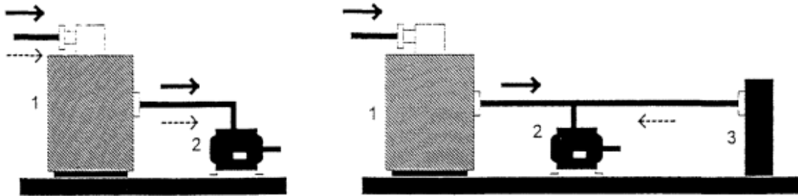
Рис. 1. Правильная компенсация реактивной мощности электродвигателя.
