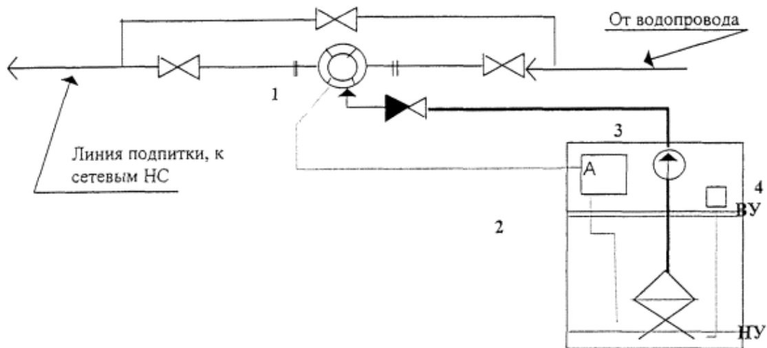
Рис 17. Схема установки для дотирования комплексонв.
