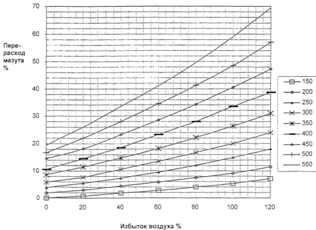
Рис. 14. Влияние избытка воздуха на перерасход мазута (справа - температура уходящих газов °С). Базовое топливо - C_4H_5 , t_{ух.газов} - 150 °С, избыточный воздух =
