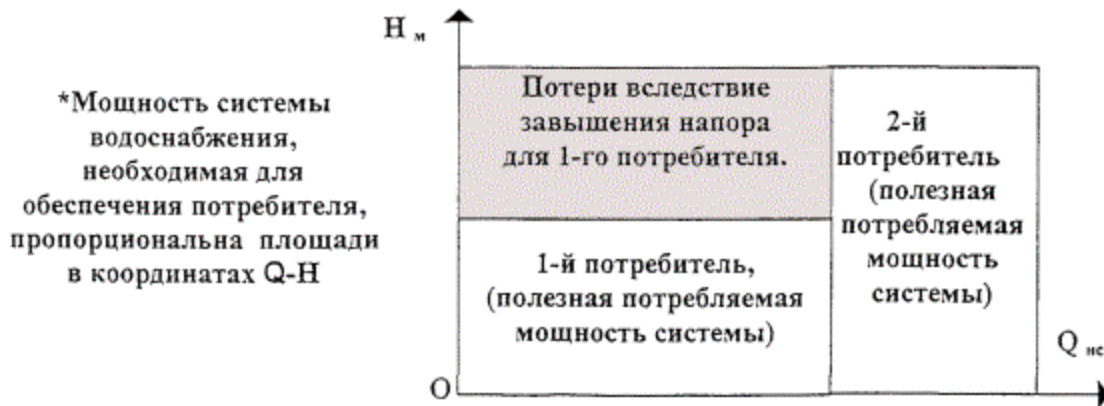
Рис. 19. Составляющие электропотребления насосами сети, работающей на двух потребителях с различным требуемым напором.
