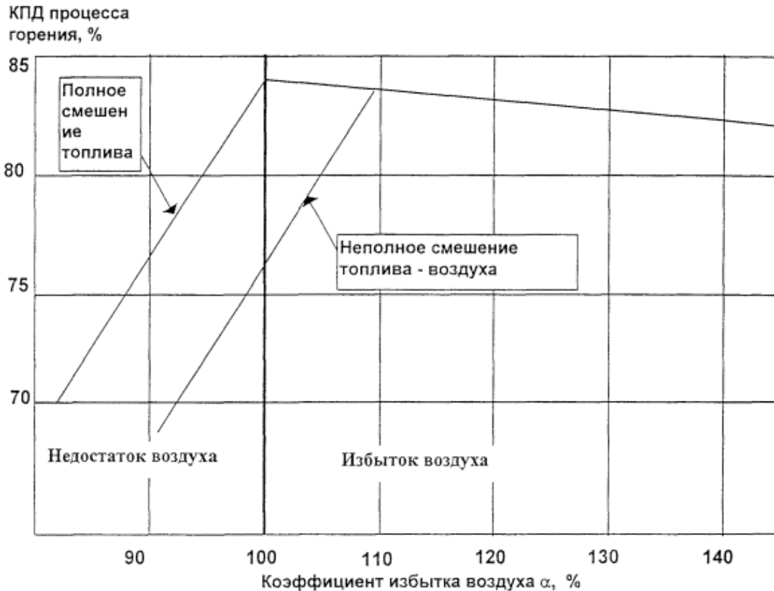
Рис 16. Влияние процессов смесеобразования и коэффициента избытка воздуха в горелочных устройствах на КПД горения газа, t_{yx} = 183^\circ\text{C} .
