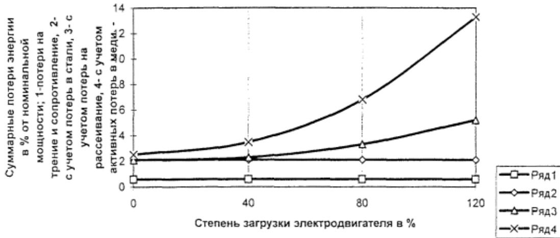
Рис. 2. Сложение составляющих потерь мощности в электродвигателях.
