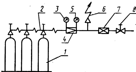
а) Ramпа с 3 и менее баллонами
