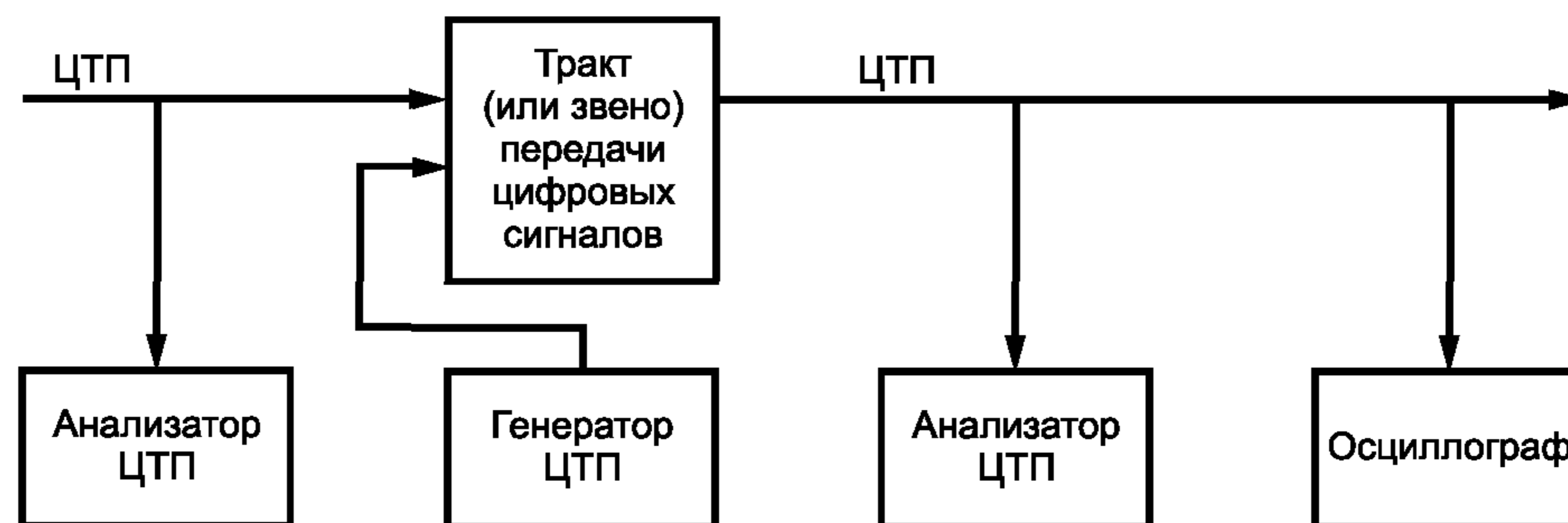
Рисунок 2 — Схема проведения измерений параметров цифрового транспортного потока
