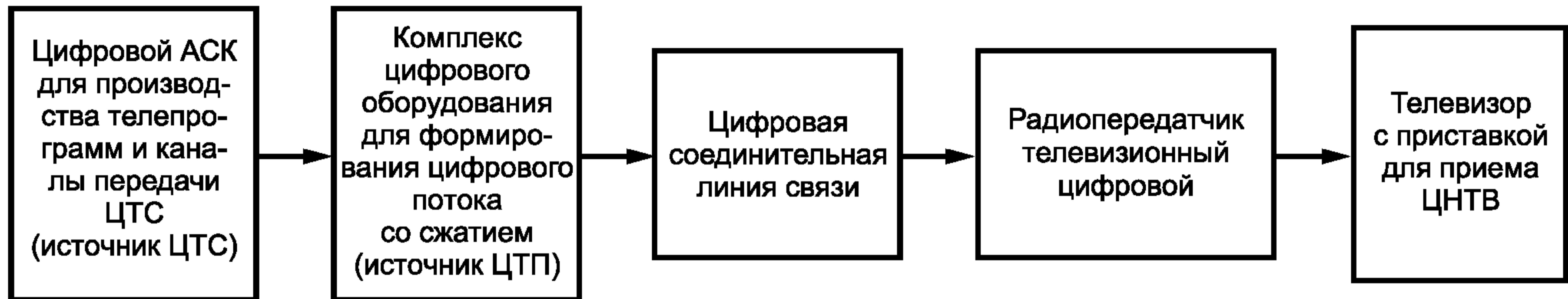
Рисунок Б.1 — Структурная схема типового тракта наземного цифрового телевидения (ЦНТВ)
