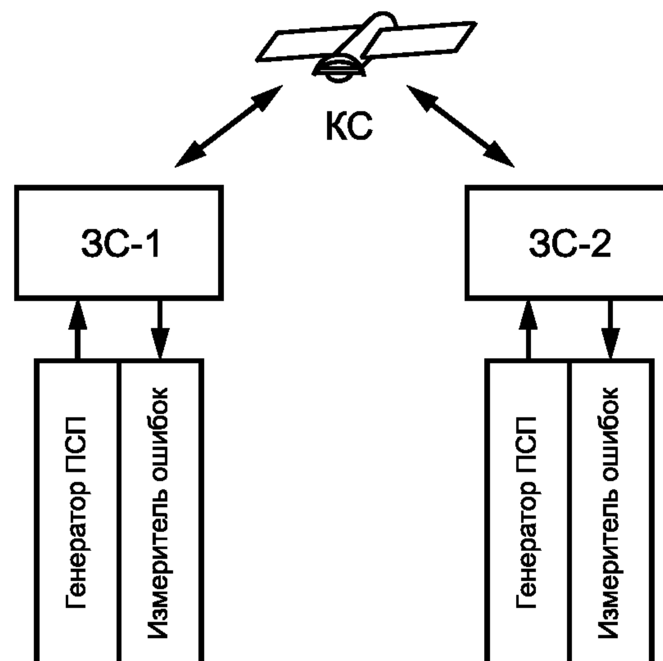
Рисунок 4.12 — Измерение показателей качества по схеме «точка — точка»
