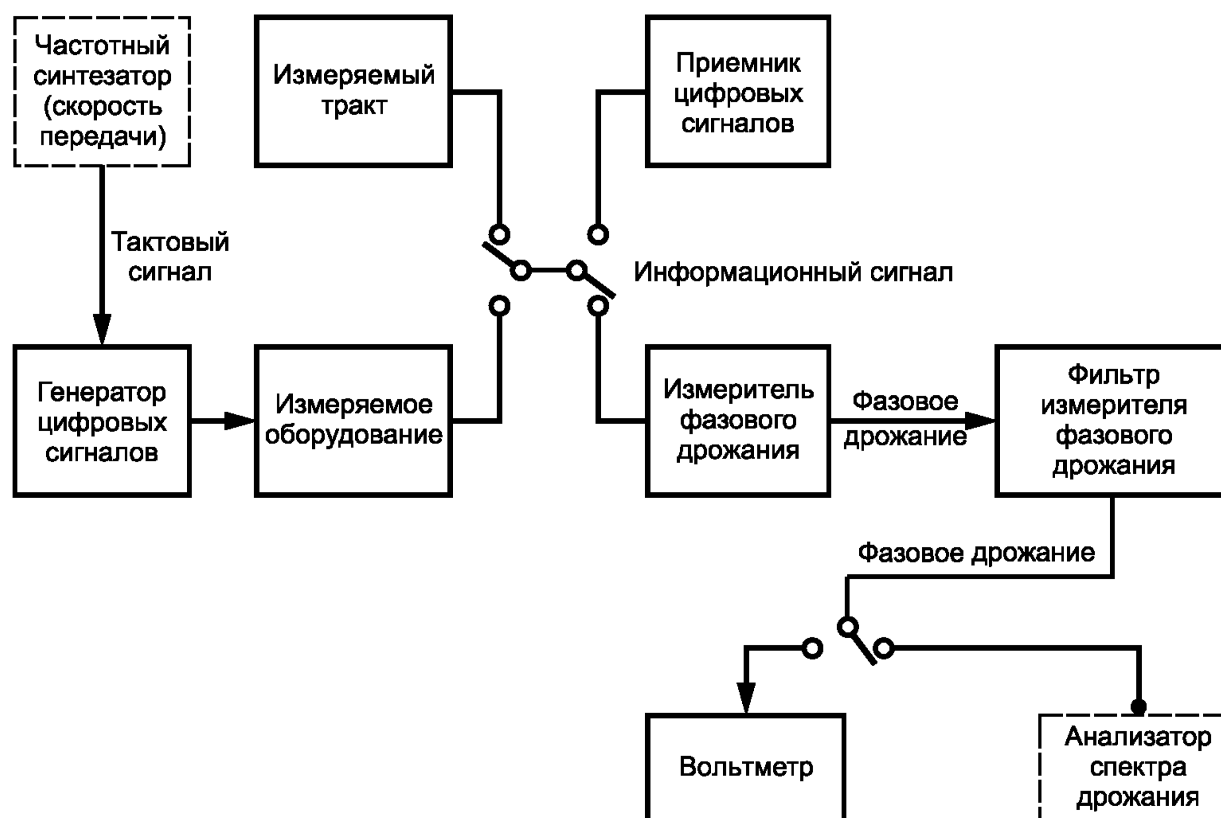
Рисунок 4.7 — Схема измерения выходного фазового дрожания
