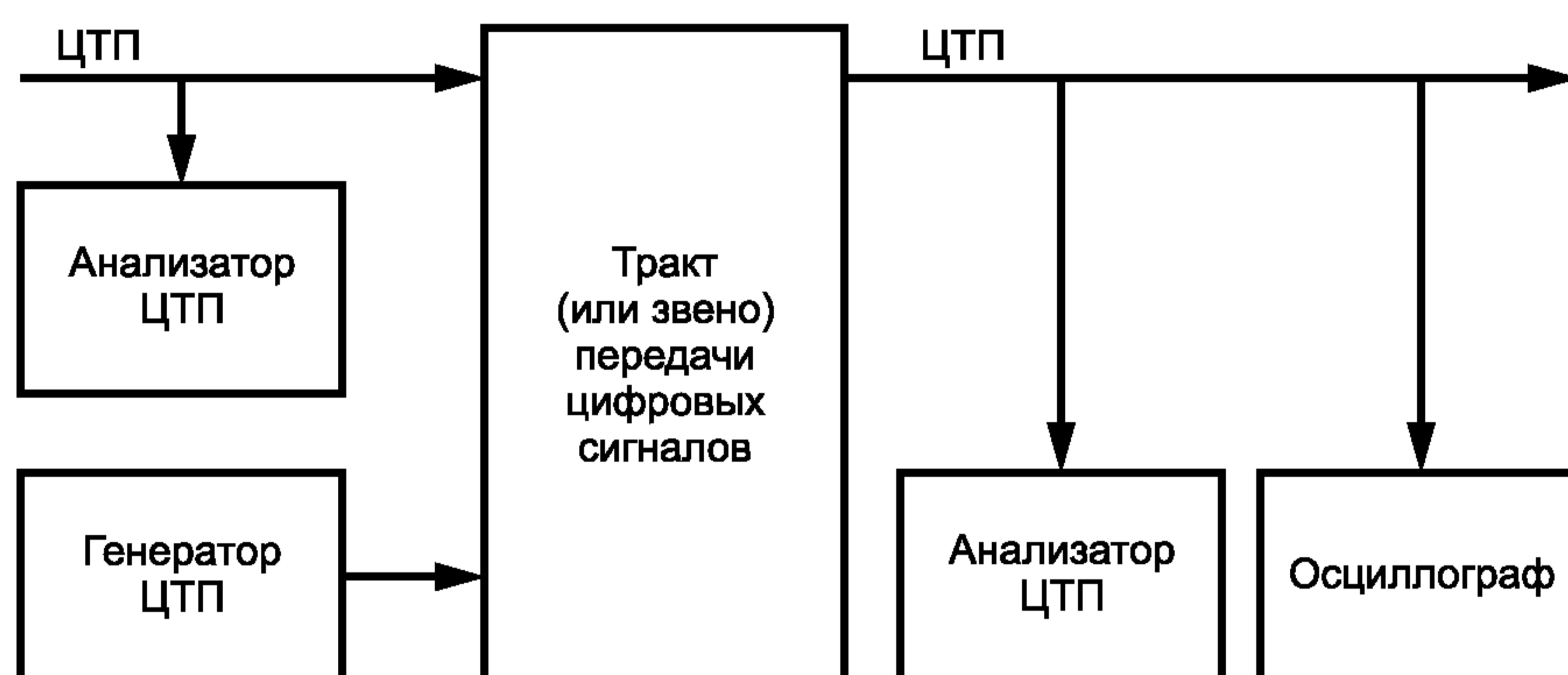
Рисунок 5.1 — Схема проведения измерений параметров цифрового транспортного потока
