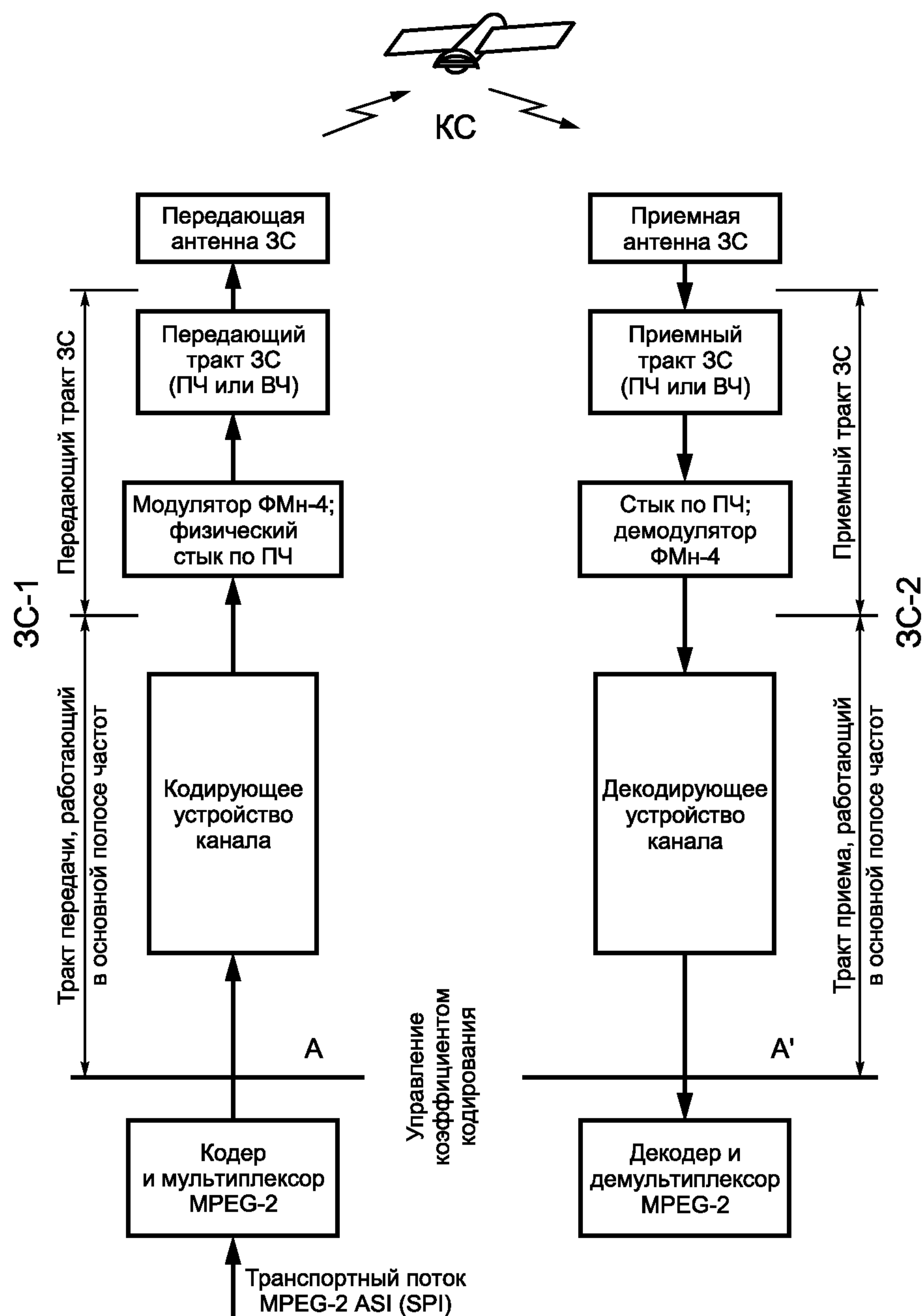
Рисунок 4.10 — Структурная схема СЛТ передачи сигналов ЦТВ
