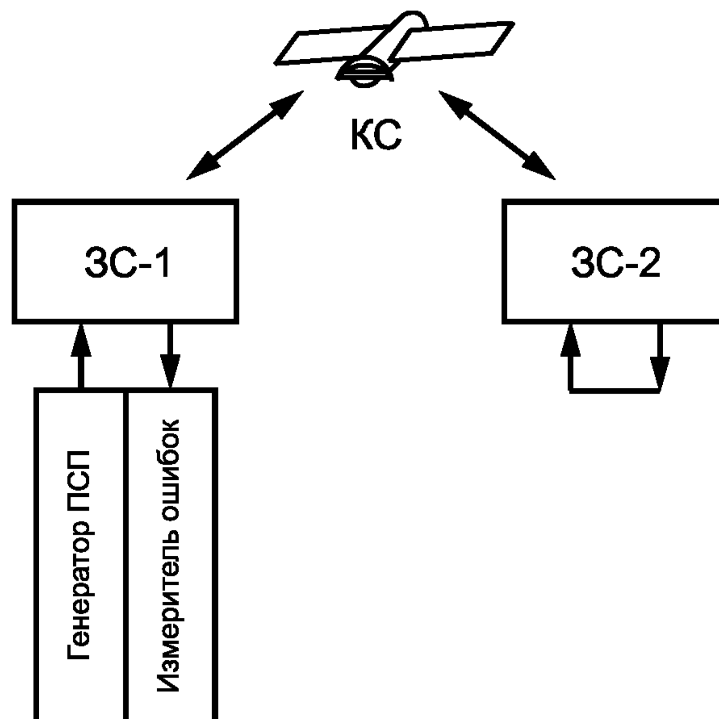
Рисунок 4.13 — Измерение показателей качества с включением шлейфа
