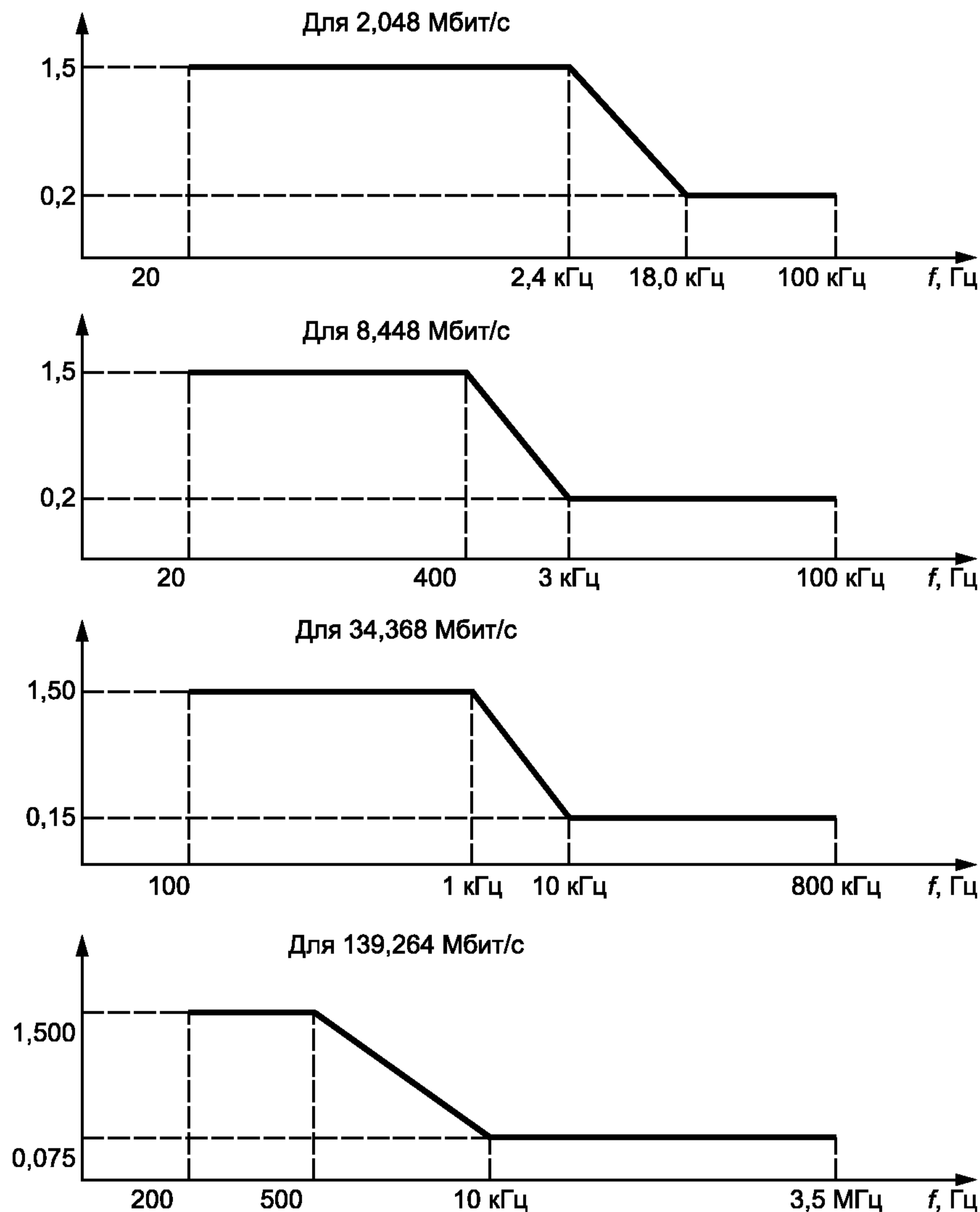
Рисунок 4.16 — Маски сигналов с предельным фазовым дрожанием
