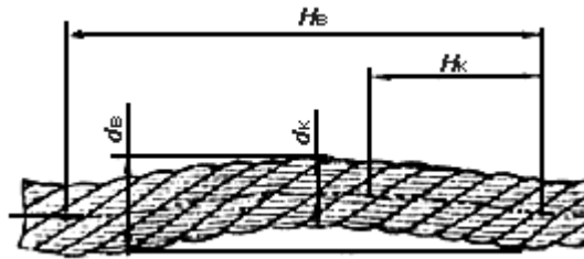
Рис.2. Волнистость каната
