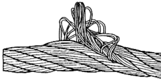
Рис.4. Выдавливание сердечника
