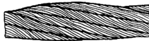
Рис.6. Местное увеличение диаметра каната
