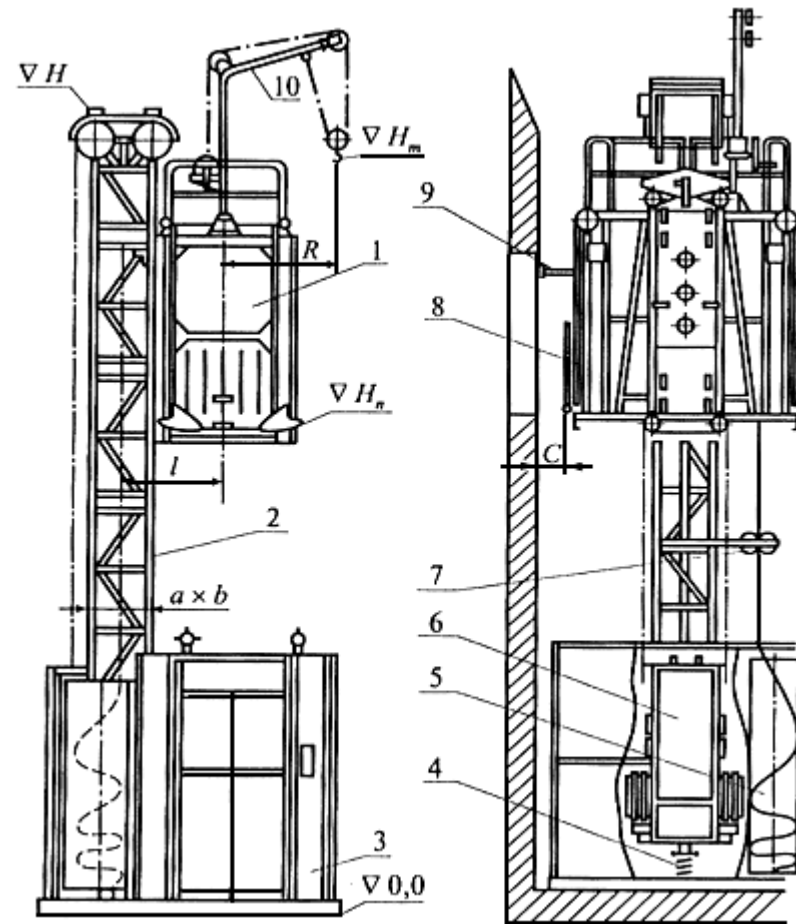
1 - кабина; 2 - мачта; 3 - опорный блок; 4 - буфер; 5 - контейнер электрокабеля; 6 - противовес; 7 - ловушка; 8 - трап; 9 - узел крепления; 10 - устройство монтажное
