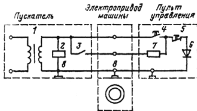
Рис. 19. Примерная схема автоматического контроля заземления передвижной машины
