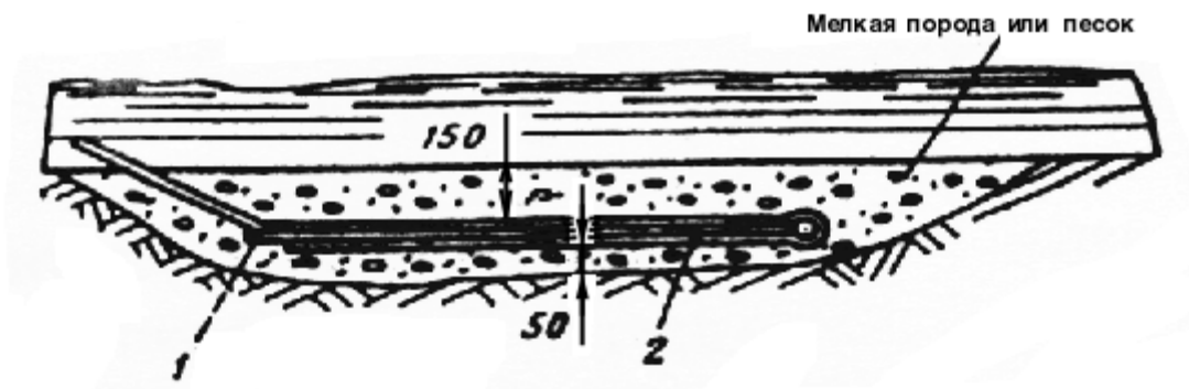
Рис. 7. Расположение заземлителя в сточной канаве:
