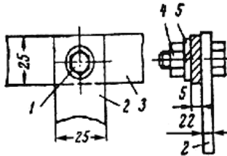
Рис. 2. Присоединение заземляющего проводника из полосовой стали к магистрали:
