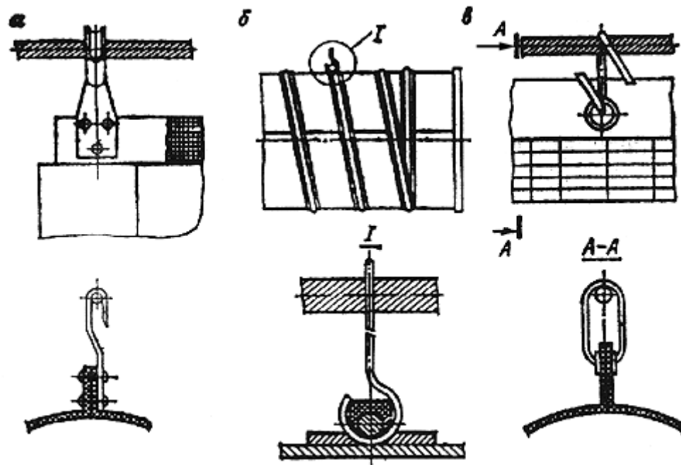
Рис. 21. Примерные схемы заземления металлических деталей гибких вентиляционных труб:
