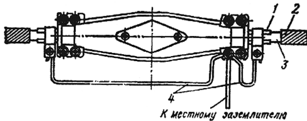
Рис. 15. Схема заземления соединительной муфты:
