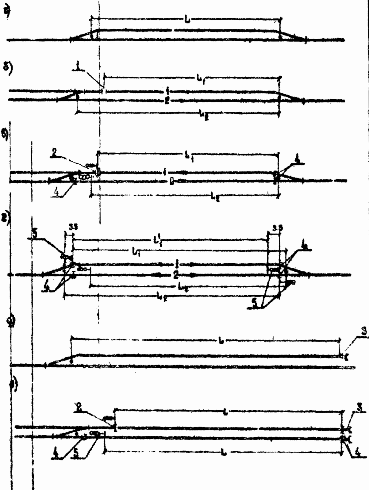
Схема 2. Полезная длина ( L ) станционных путей с учетом расположения стрелов и изолирующих стыков.
