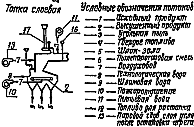
Рис. 8.2. Технологическая схема сушильной установки (кипящий слой) с различными типами топочных устройств
