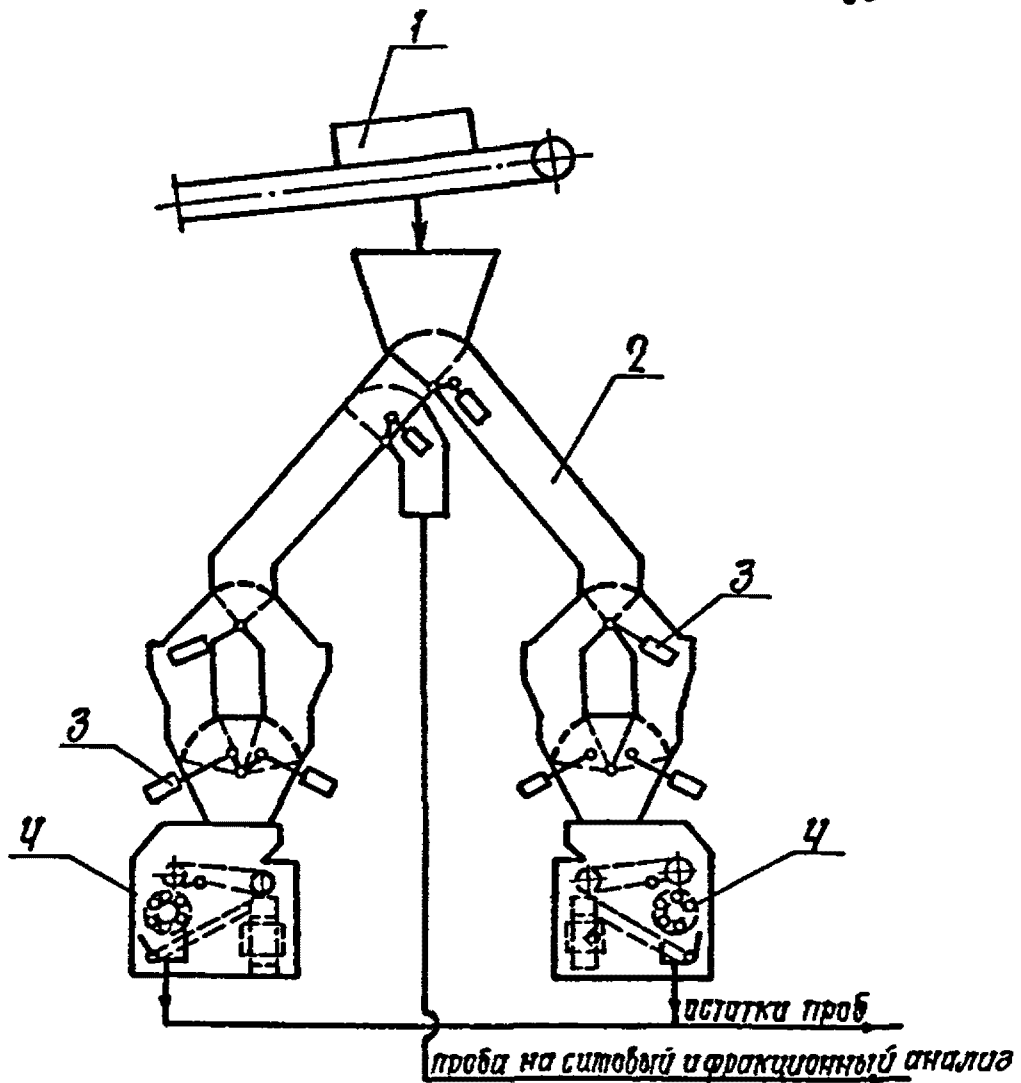
Технологическая схема пункта централизованного отробования для фабрик, обогащающих коксующиеся угли
