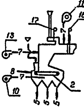
Рис. 8.3. Технологическая схема сушильной установки (труба-сушилка) в различных типах топочных устройств.
