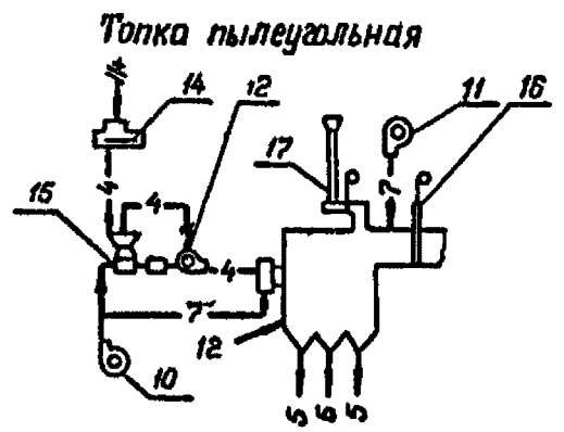
Рис. 8.3. Технологическая схема сушильной установки (труба-сушилка) в различных типах топочных устройств.
