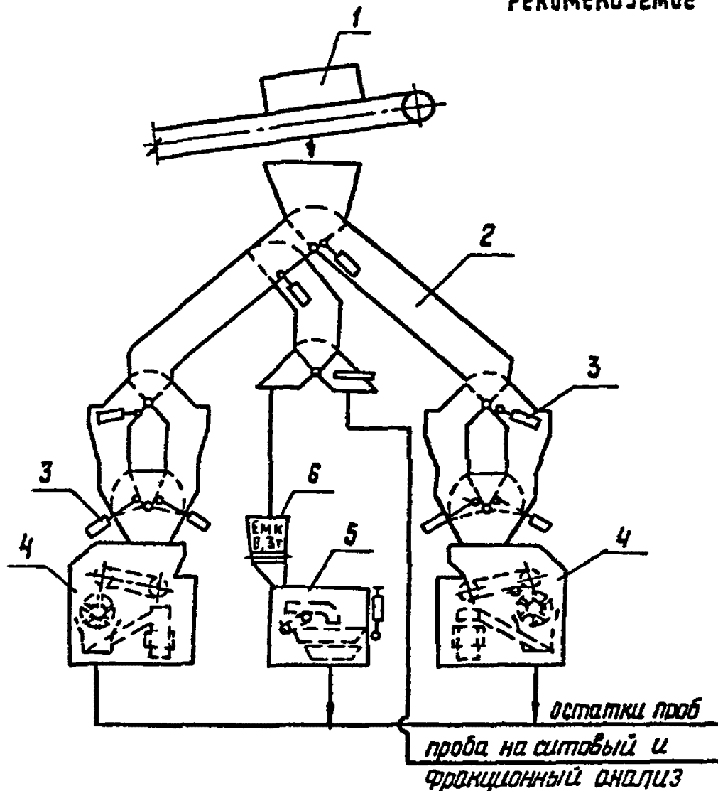
Технологическая схема пункта централизованного отпробования для фабрик, обогащающих энергетические угли и антрациты.
