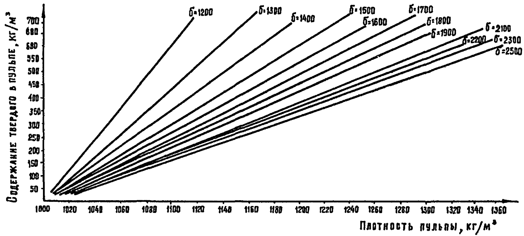
Рис.77. Зависимость плотности пульпы от содержания твердого при различной его плотности - б [кг/м³]
