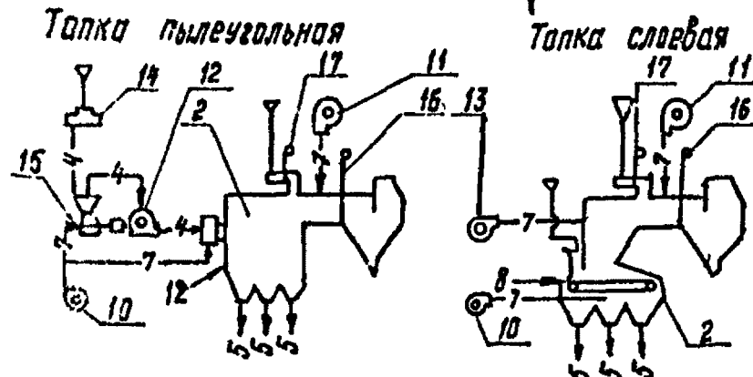
Рис. 8.1. Технологическая схема сушильной установки (барабанная сушилка) с различными типами топочных устройств.
