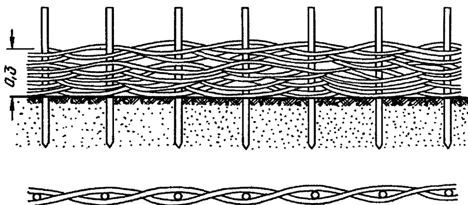
Рис. 8. Плетневая стенка
