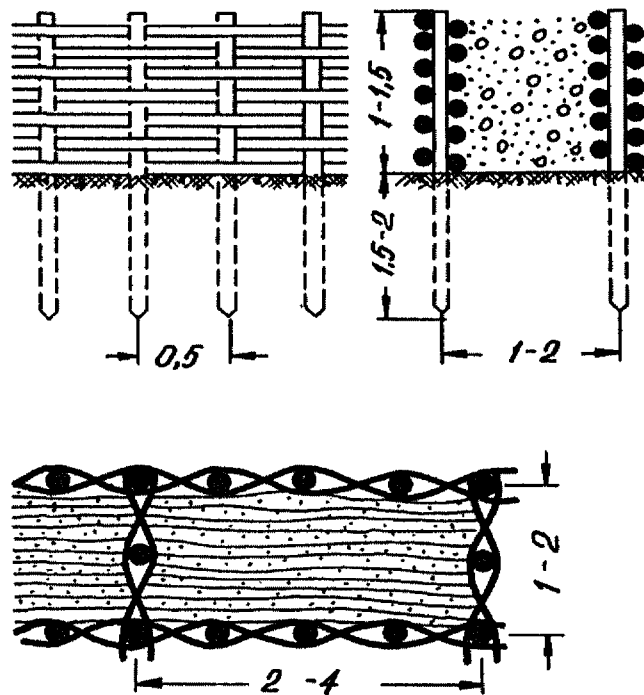
Рис. 11. Двухрядный плетень
