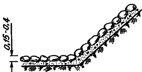
Рис. 3. Мощение камнем
