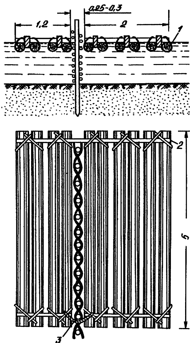
Рис. 10. Плот для устройства плетня: 1 — неокоренные еловые бревна диаметром 0,2; 2 — жердь диаметром 0,1; 3 — чалка диаметром 0,02
