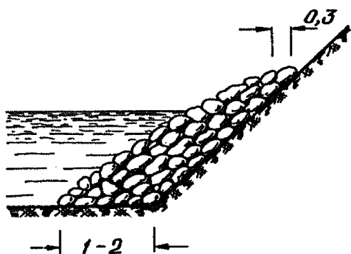
Рис. 1. Каменная наброска (средняя толщина наброски 0,65—1 м)
