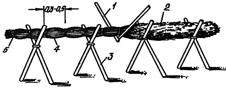
Рис. 12. Вязка хвостяного каната: 1 — сжим; 2 — хвост; 3 — козлы; 4 — канат; 5 — перевязка
