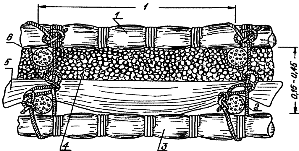
Рис. 9. Хворостяной тюфяк (разрез): 1 — верхний канат верхней сетки; 2 — верхний канат нижней сетки; 3 — нижний канат нижней сетки; 4 — верхний слой хвороста; 5 — нижний слой хвороста; 6 — нижний канат верхней сетки
