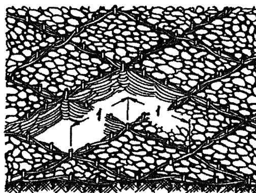
Рис. 2. Каменная наброска в плетневые клетки
