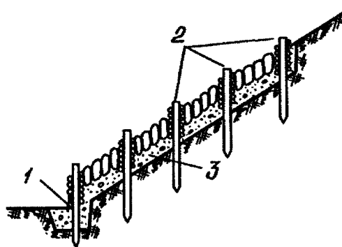
Рис. 4. Мощение в плетневых клетках: 1 — плетневая заборка; 2 — плетень; 3 — слой щебня
