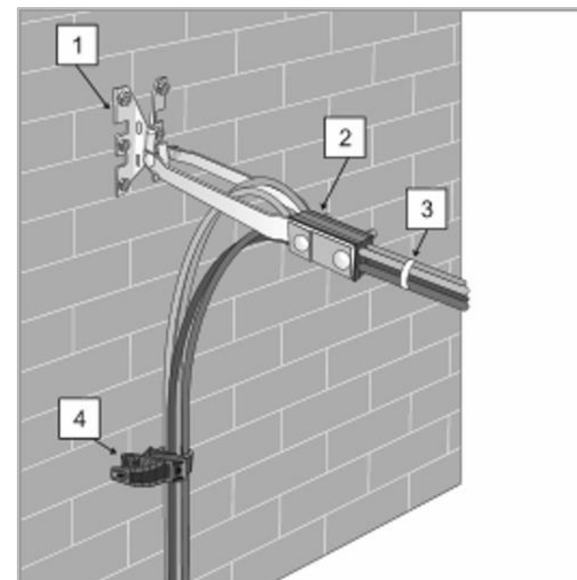
Рисунок 2 Крепление СИП-4 к стене здания
